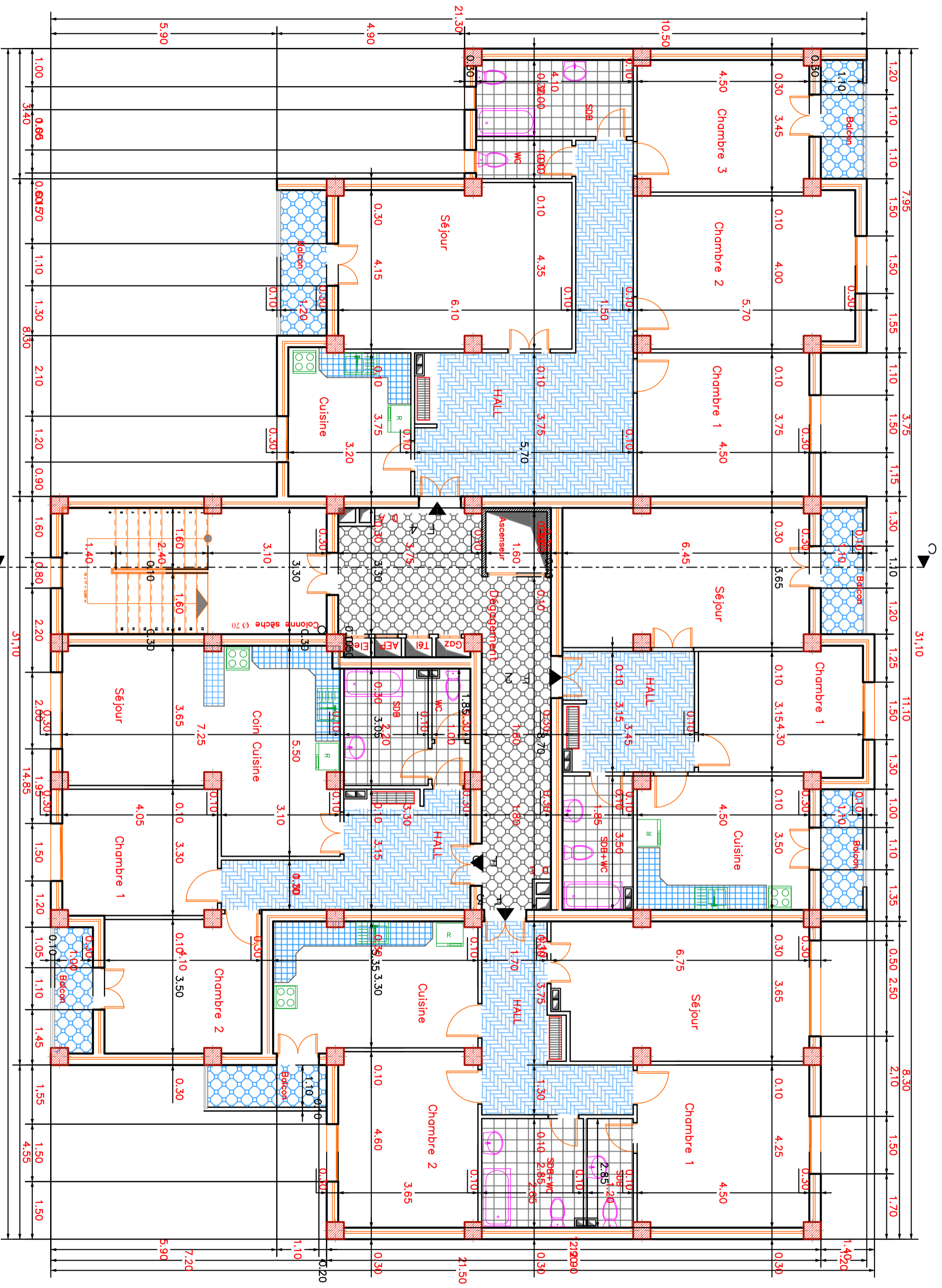
PLAN ETAGE COURANT(2,3,4,5,6,7,8,9 et 10 )
