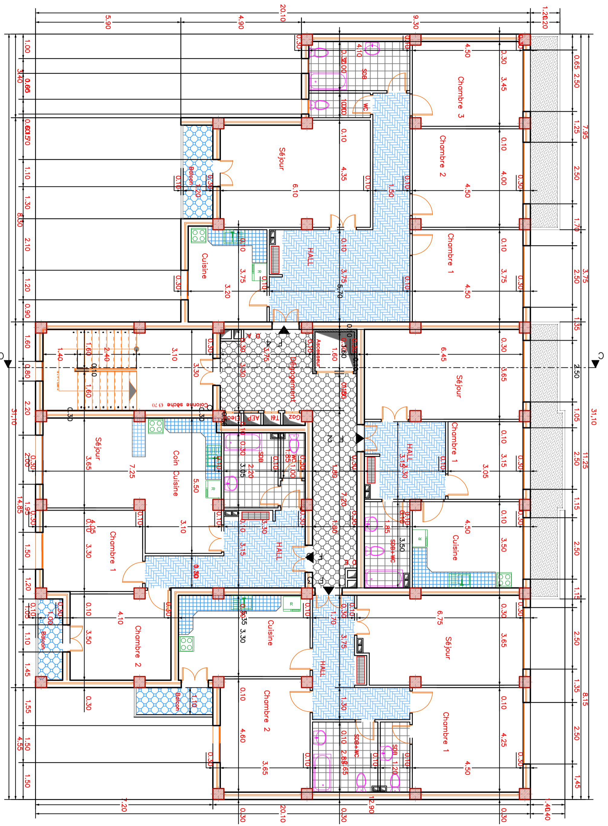
PLAN ETAGE 11
