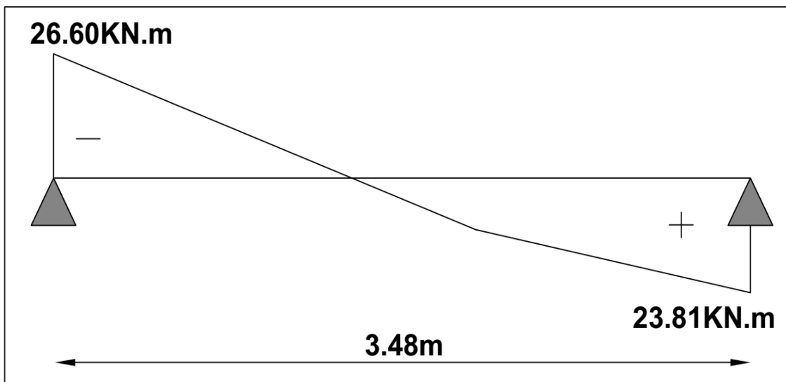
Figure III.32: Diagrammes des efforts tranchants et des moments fléchissant
