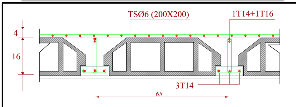
Figure III.15: schéma de ferrailage de plancher RDC.
