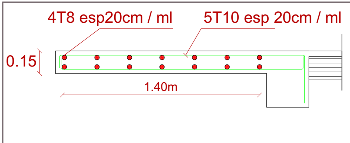
Figure III.6: Schéma du ferrailage des balcons.
