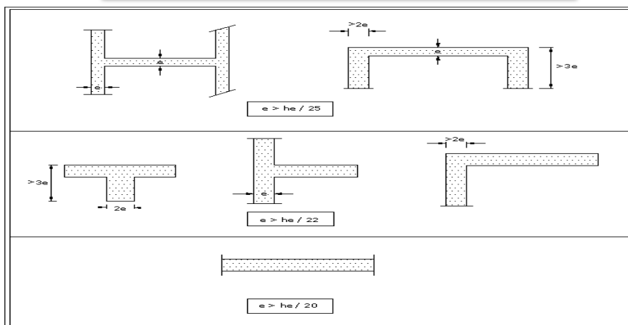
Figure II.4: coupe de voile en plan
