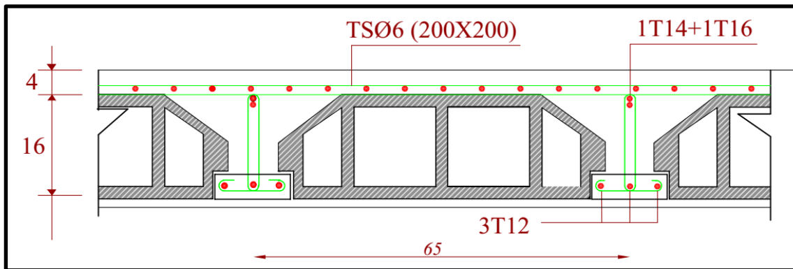
Figure III.14: schéma de ferrailage de plancher étage courant et terrasse.
