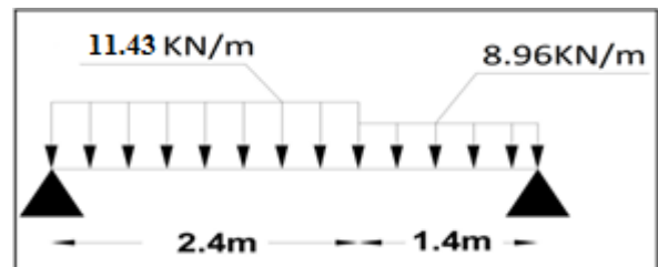
Figure III.22: Schéma statique des escaliers
