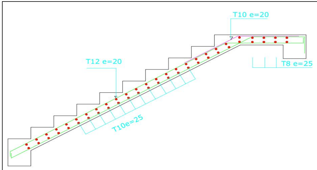
Figure III.34: Schéma de L'escalier de sous-sol.
