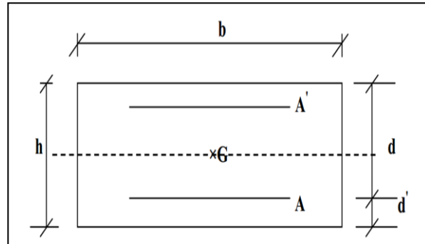
Figure (III.29) : Section de calcul de contrainte.
