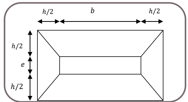
Figure VI.4: Schéma de transmission des charges.
