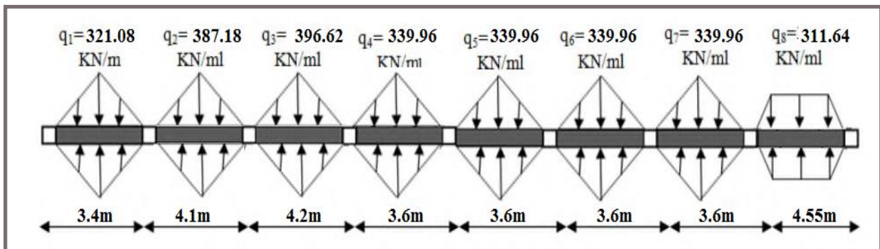
Figure VI.9: Charges transmises aux nervures longitudinales de radier.
