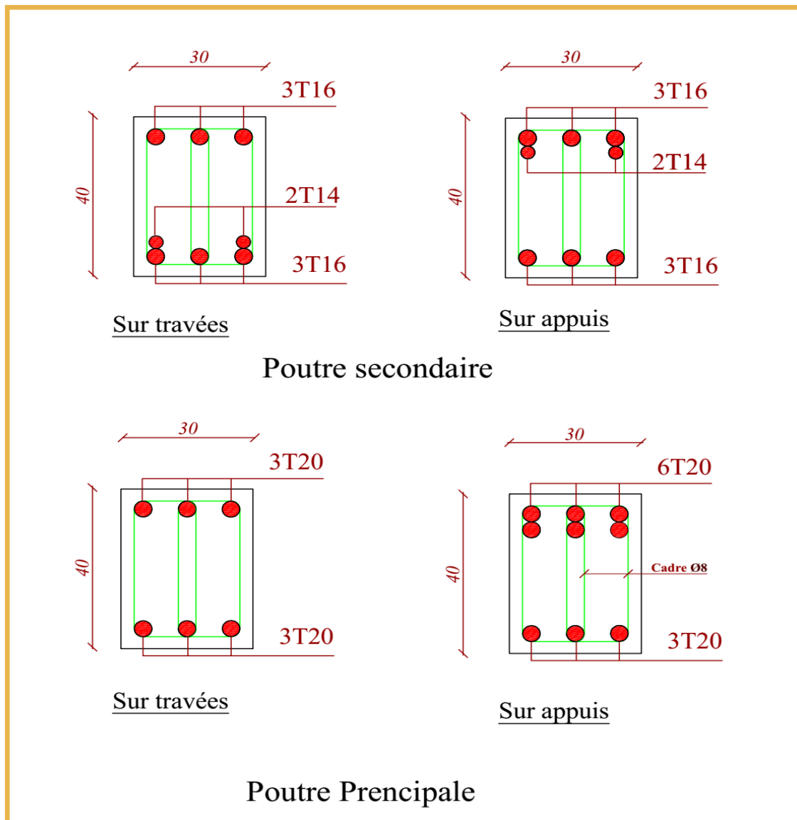
Figure.V.2: Schémas de ferraillage des poutres.
